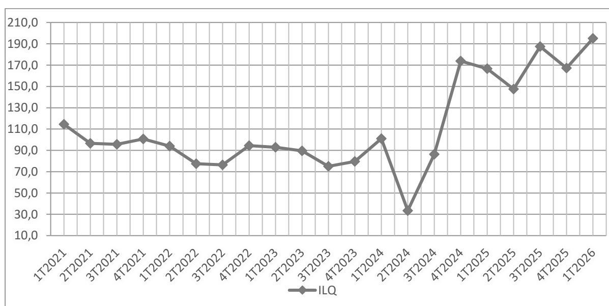
Graphique 3 : Evolution de l'Indice Laspeyres des Quantités (ILQ) à l'Exportation
