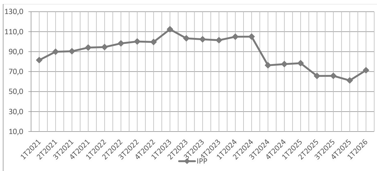
Graphique 2 : Evolution de l'Indice Paasche des Prix (IPP) à l'Exportation
