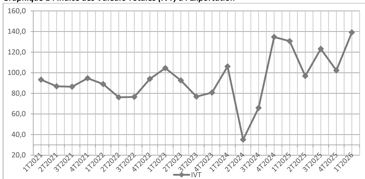
Graphique 1 : Indice des Valeurs Totales (IVT) à l'Exportation
