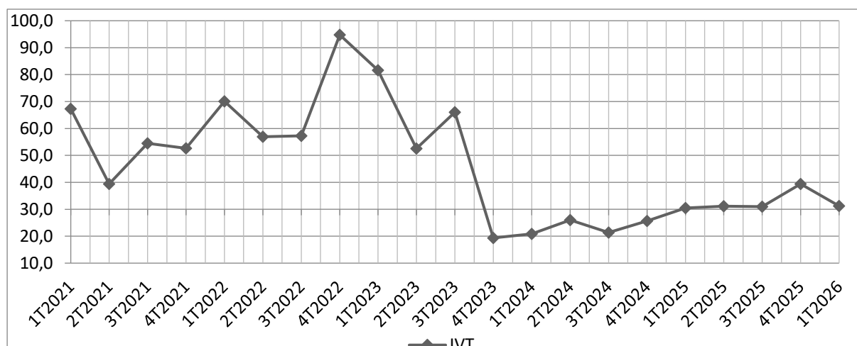
Graphique 4 : Évolution de l'Indice des Valeurs Totales (IVT) à l'Importation
