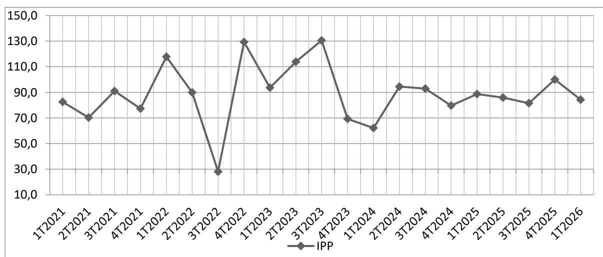
Graphique 5 : Évolution de l'Indice Paasche des Prix (IPP) à l'Importation
