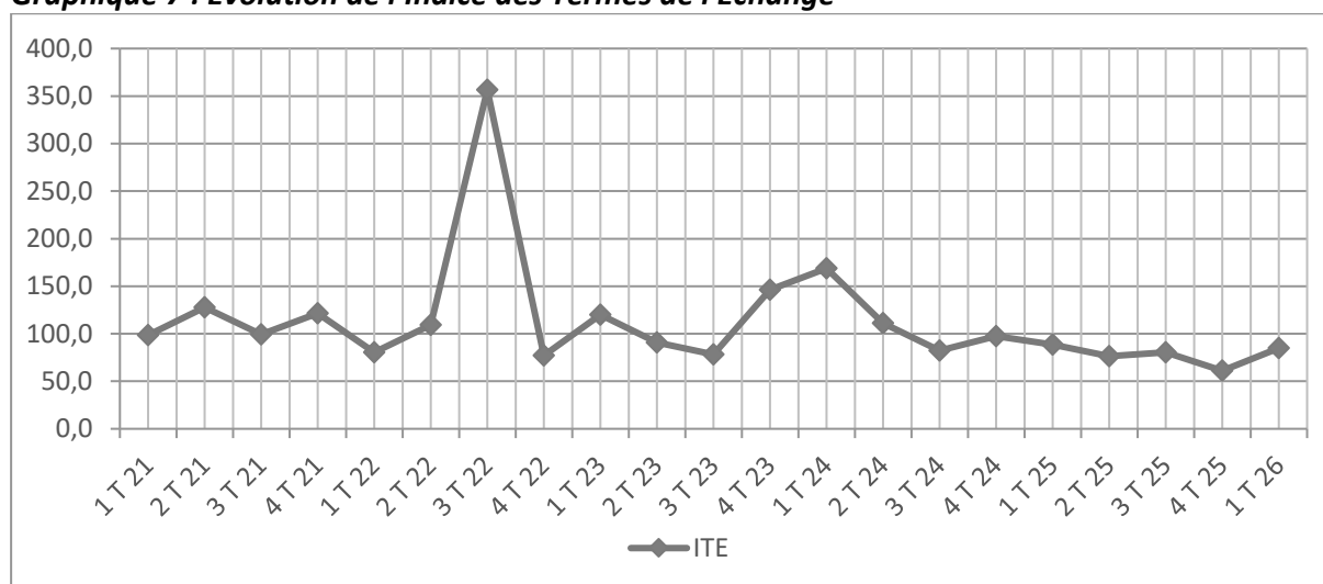
Graphique 7 : Évolution de l'Indice des Termes de l'Echange
