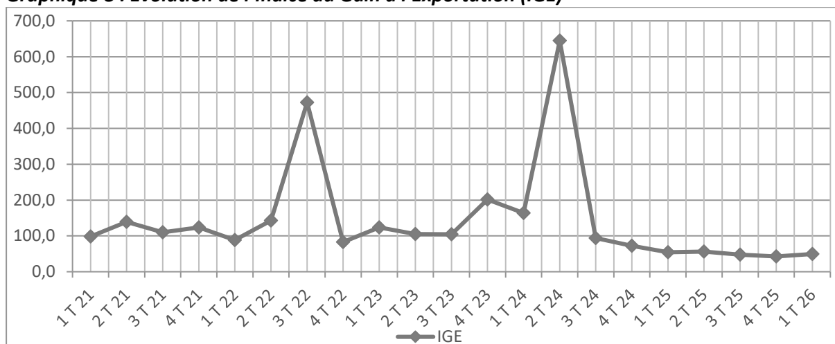
Graphique 8 : Évolution de l'Indice du Gain à l'Exportation (IGE)
