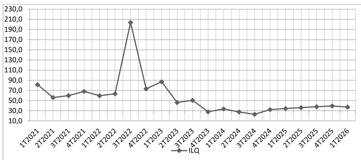
Graphique 6 : Évolution de l'Indice Laspeyres de Quantité (ILQ) à l'Importation
