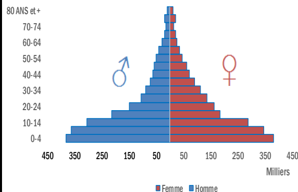
Pyramide des âges de la population de Tahoua en 2017
